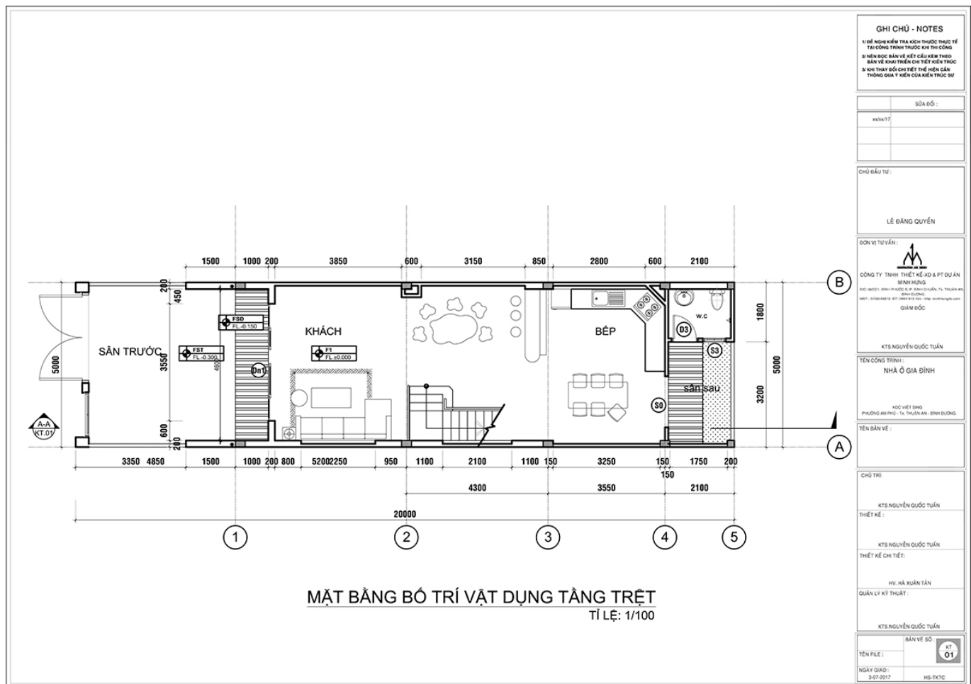
Mặt Bằng Trệt.
