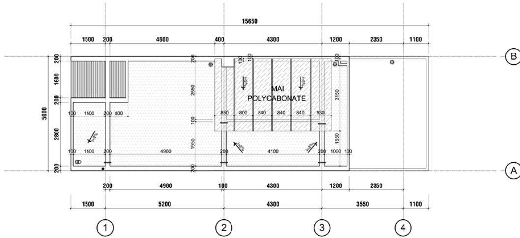
MẶT BẰNG MÁI TỈ LỆ: 1/100
