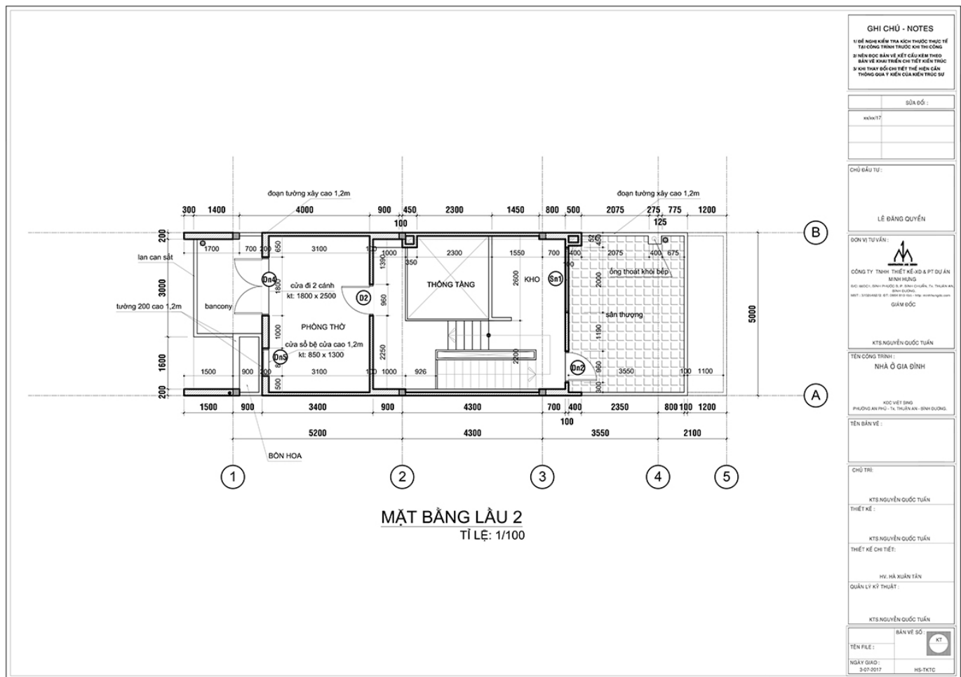
Mặt Bằng Lầu 2.
