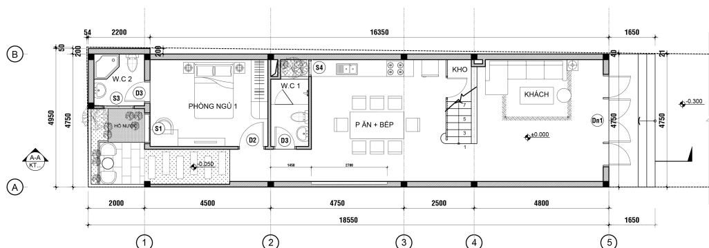
MẶT BẰNG TẦNG TRỆT TỈ LỆ: 1/50
